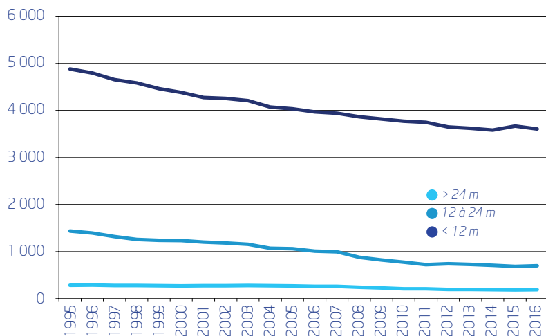
Évolution du nombre de navires de pêche en métropole
